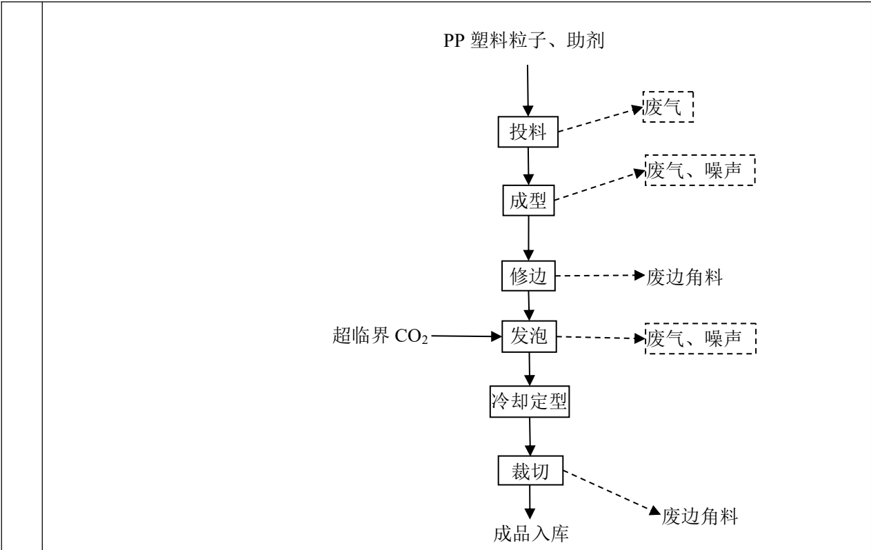
图2-10 项目生产工艺流程图
