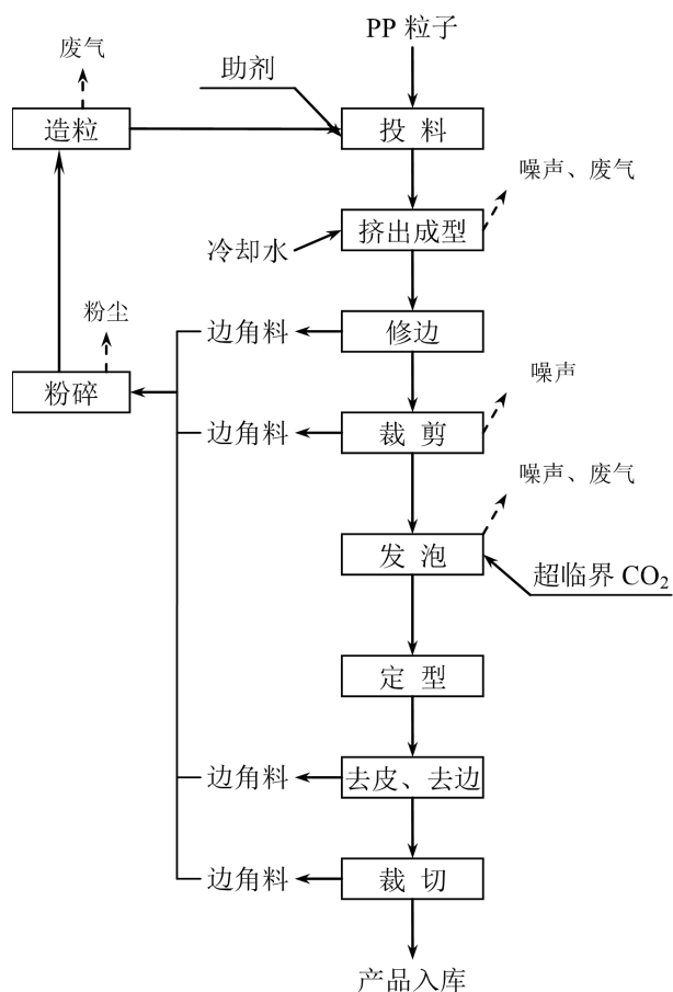
图 2-4 企业聚丙烯微孔发泡材料生产工艺及污染物产生示意图
