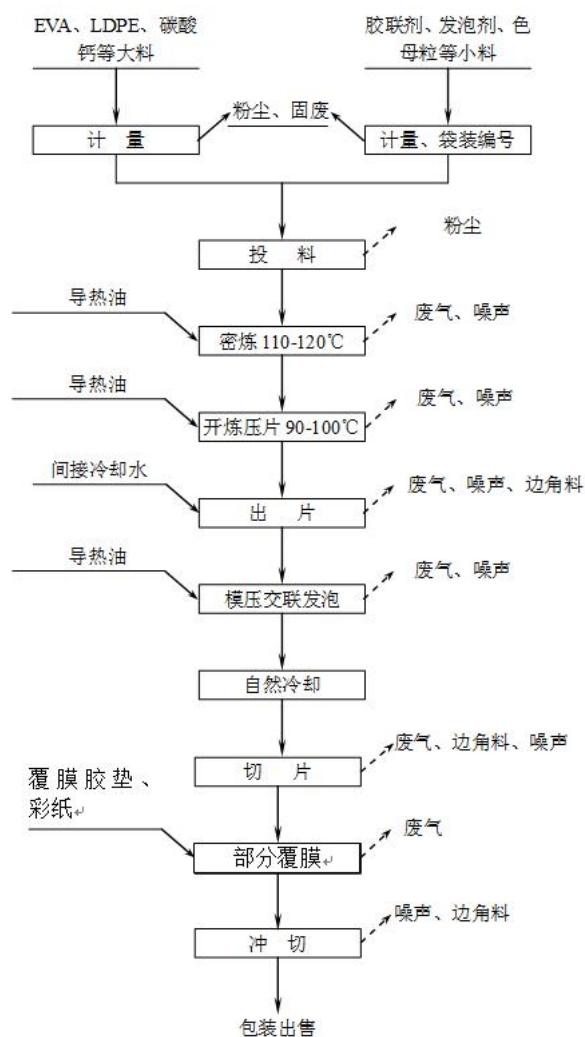
图 2-5 企业 EVA 泡沫地垫生产工艺及污染物产生示意图
