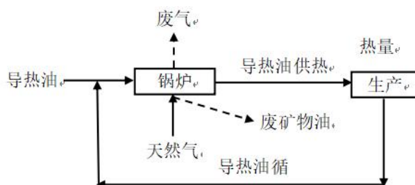
图 2-9 工艺流程及污染物产生示意图
