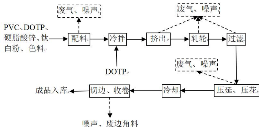
图2-8 3C电子屏幕缓冲膜工艺流程及污染物产生示意图
