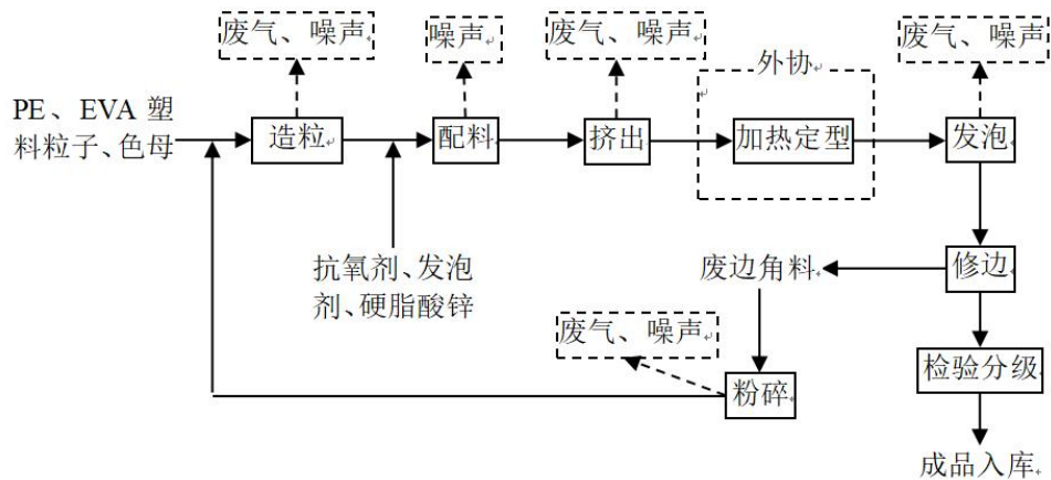
图 2-6 企业 IXPE 板材生产工艺及污染物产生示意图
