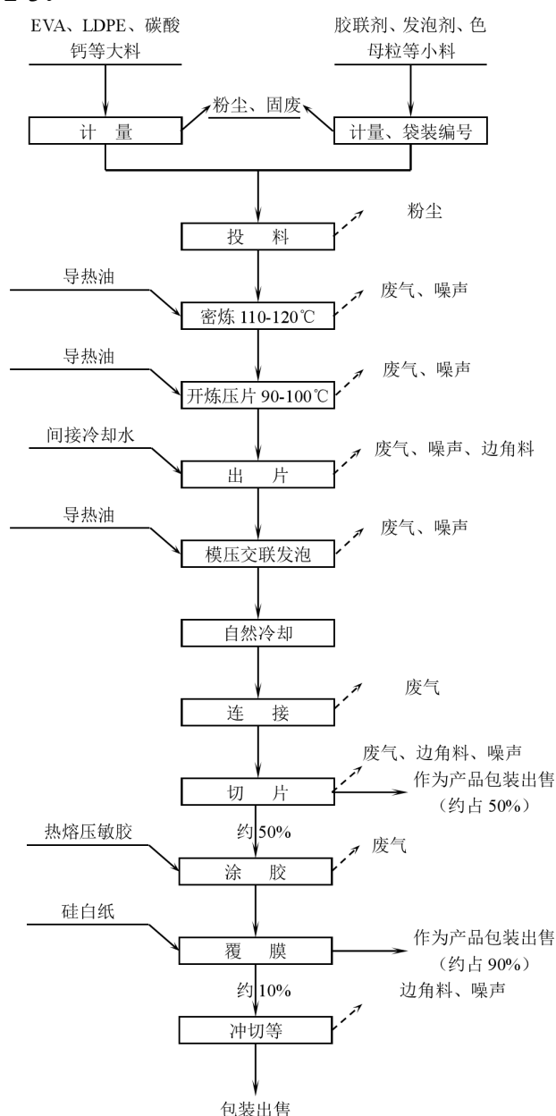
图 2-3 企业 EVA 发泡材料工艺流程及污染物产生示意图
