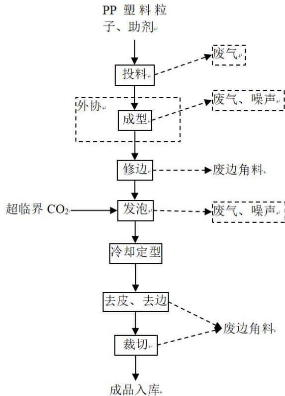
图 2-7 5G 微波天线罩工艺流程及污染物产生示意图
